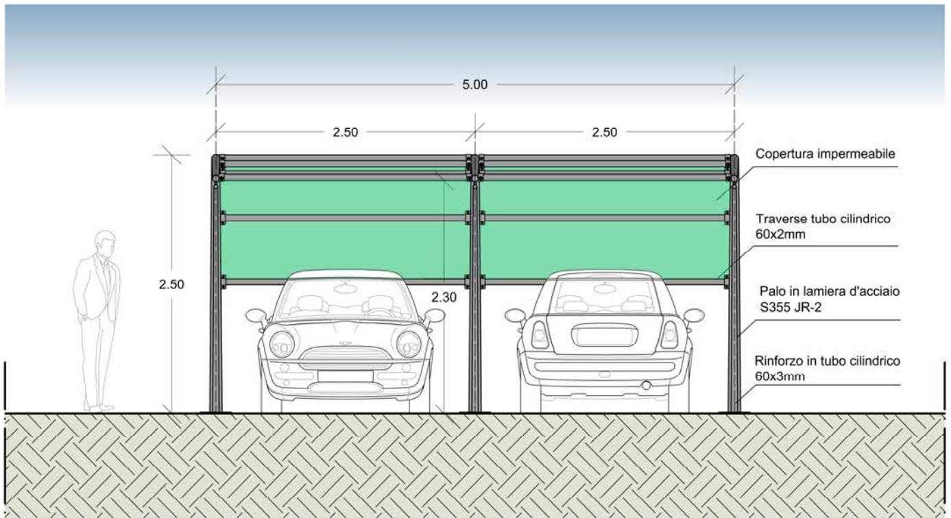
PROSPETTO FRONTALE
