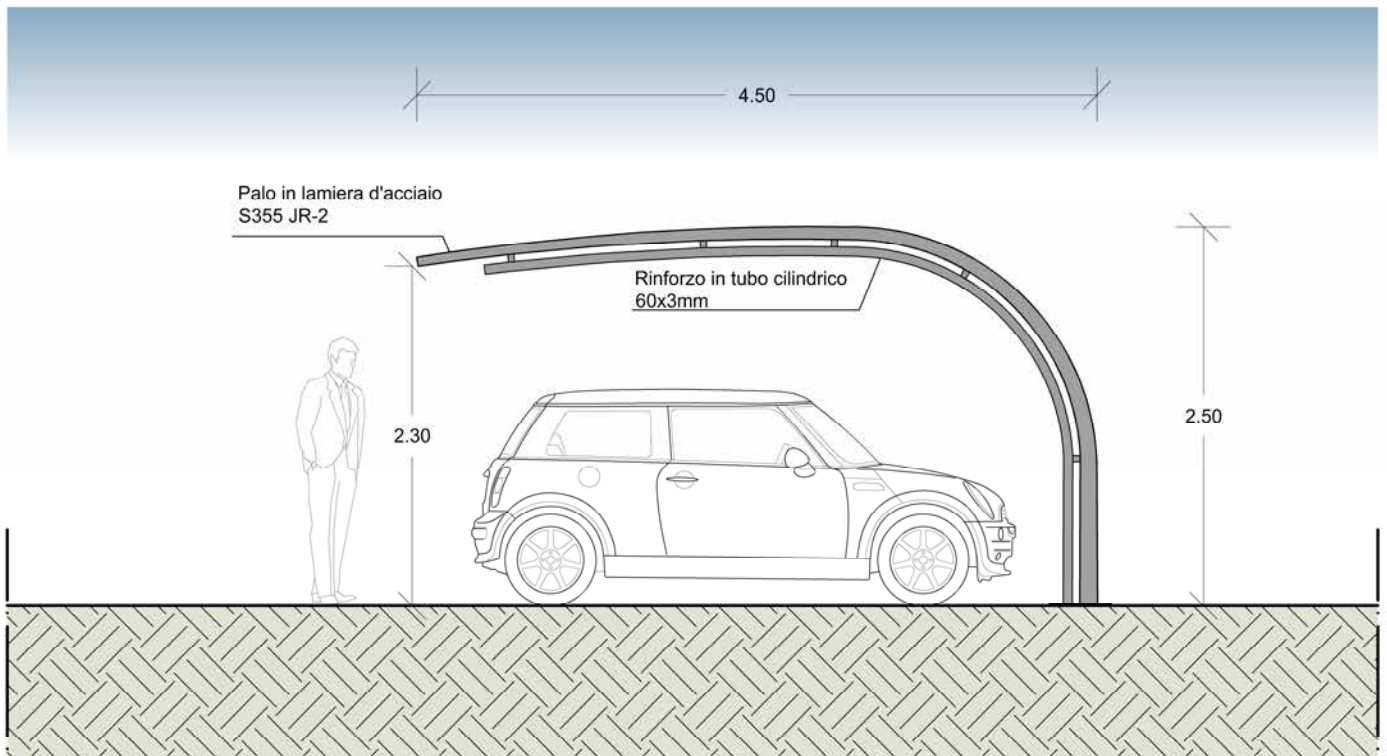
PROSPETTO LATERALE
